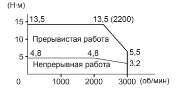
R88M-G1K020T (1 кВт)
