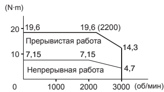
R88M-G1K520T (1,5 кВт)
