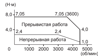
R88M-G1K520T (1,5 кВт)
