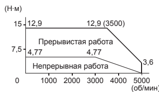
R88M-G1K530T (1,5 кВт)
