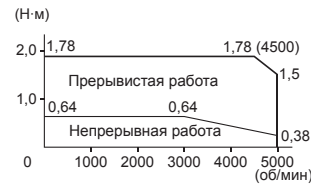
R88M-G1K530T (1,5 кВт)
